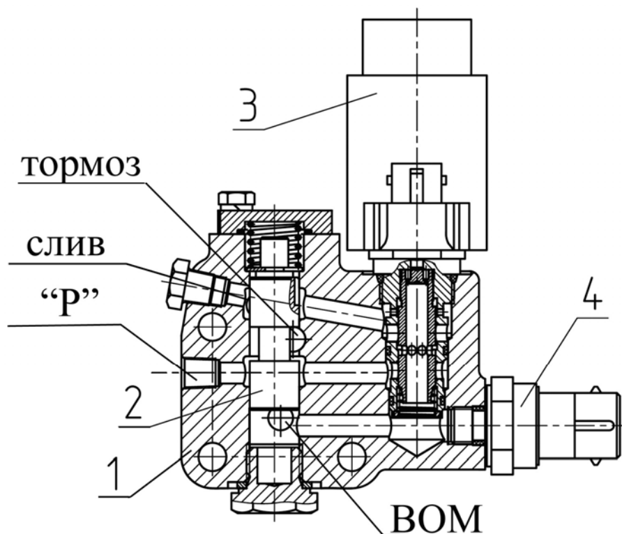
Рис. 28 Распределитель управления задним ВОМ: 1 – корпус; 2 – золотник; 3 – клапан пропорциональный; 4 – датчик давления.
