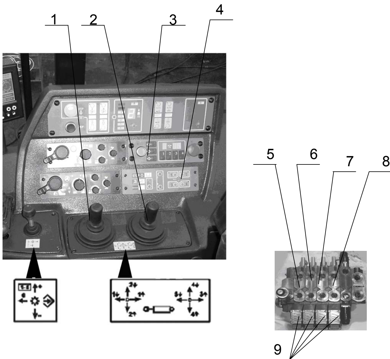
Рис.17 Правый боковой пульт кабины трактора и секционный распределитель 1 — джойстик управления секциями 7 и 8 распределителя EHS; 2 — джойстик управления секциями 5 и 6 распределителя EHS; 3 — блок программирования последовательности операций (БПО ГНС) управления секциями распределителя EHS; 4 — панель электронная комбинированная (ПЭК) систем управления двигателем и внешними потребителями ГНС; 5 — секция №4 распределителя EHS; 6 — секция №3 распределителя EHS; 7 — секция №2 распределителя EHS; 8 — секция №1 распределителя EHS; 9 — сигнализаторы неисправностей работы секций распределителя EHS.
