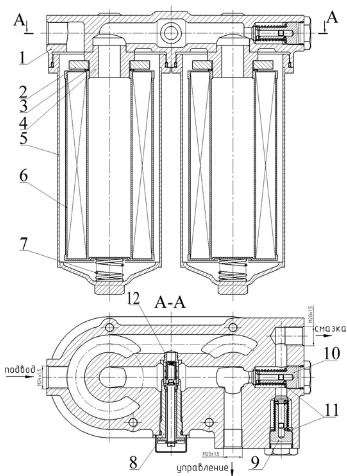
Рис. 26 Фильтр сдвоенный:
