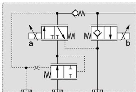
Рис.6 Электрогидравлический регулятор EHR-5LS
