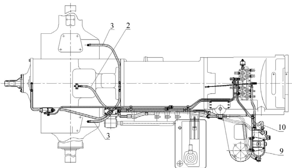
Рис. 25 Расположение элементов гидросистемы смазки трансмиссии со сдвоенным фильтром (вид сверху):
