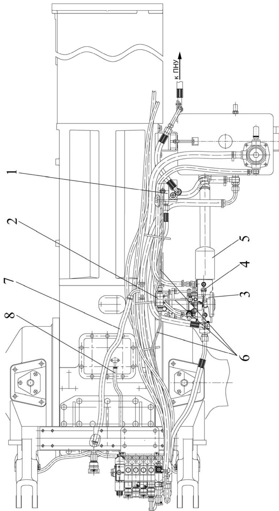
Рис.10 Компонновка узлов гидросистемы на тракторе (вид сверху): 1- электрогидравлический регулятор управления ПНУ; 2- клапан «ИПИ»; 3- насос регулируемый А10СN045; 4- датчик засоренности; 5- фильтр фирмы «Donaldson»; 6 – магистраль канала управления; 7 - магистраль свободного слива (заднего); 8- магистраль дренажная гидроцилиндров.
