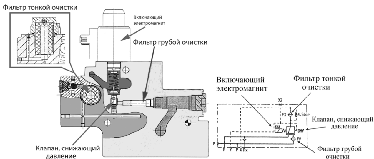
Рис.5 Схема управления рабочими секциями EHS с трехходовым редукционным клапаном
