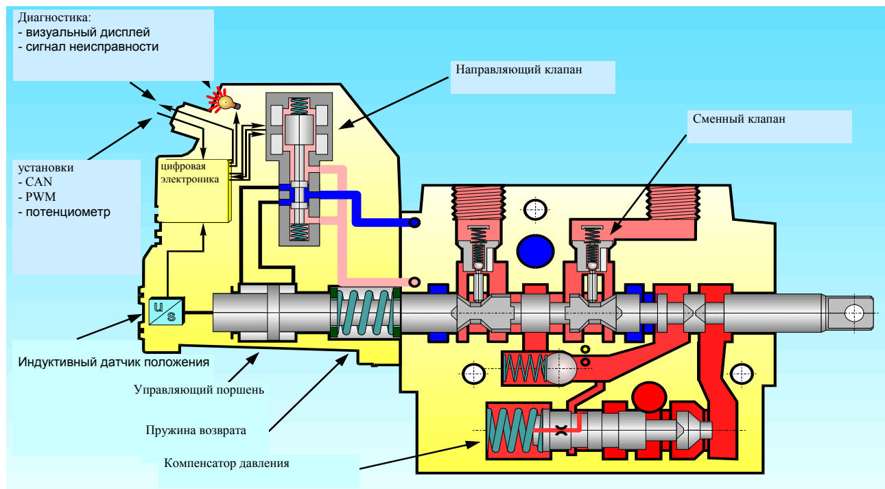
Рис.2. Схема устройства распределительной секции EHS
