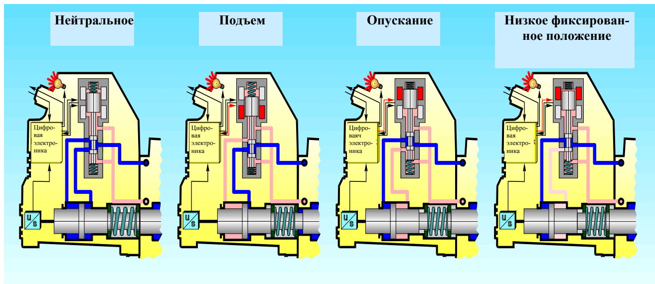
Рис.3. Схема позиционирования направляющего клапана и центрального золотника при реализации функций
