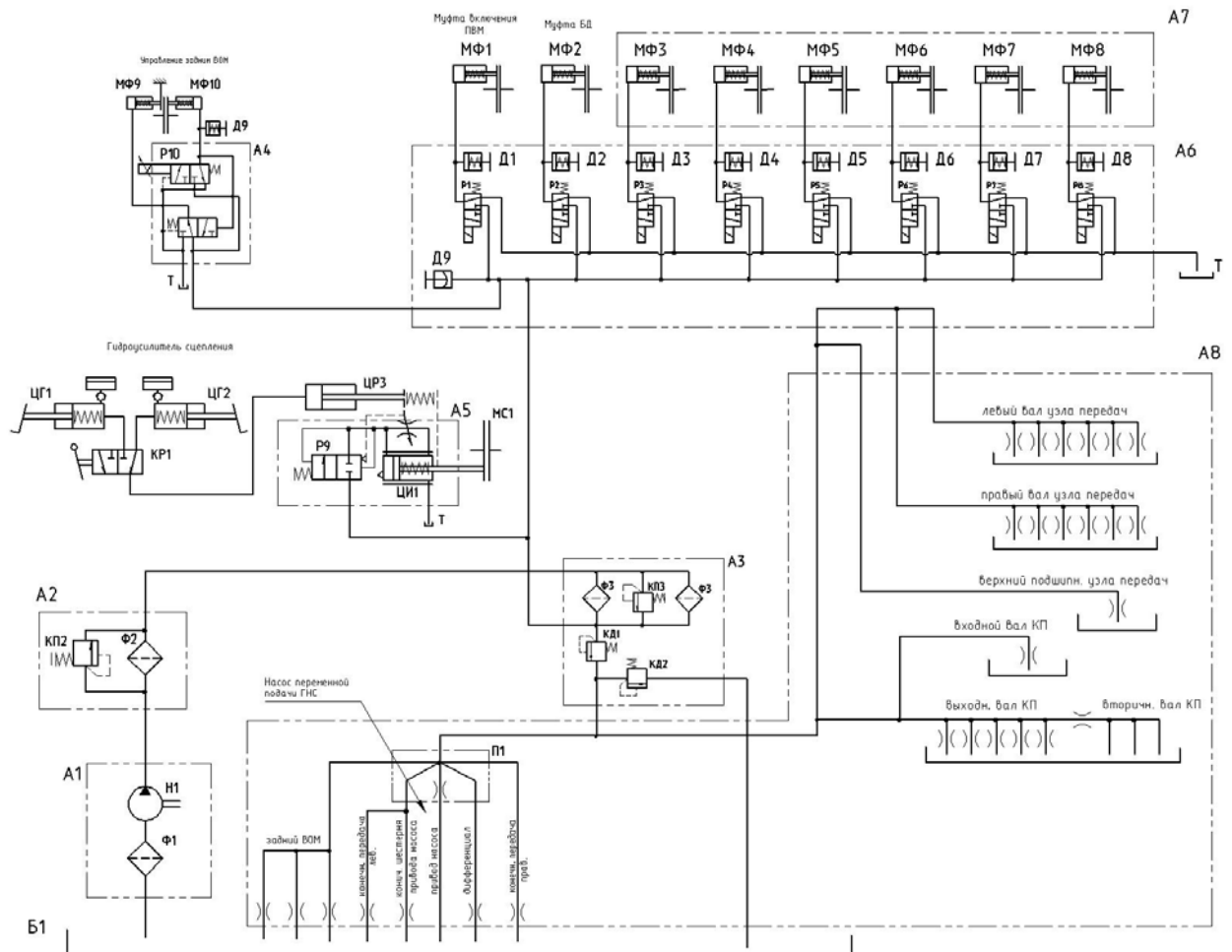
Рис. 23 Схема гидравлическая принципиальная трансмиссии со сдвоенным Фильтром и распределителем
