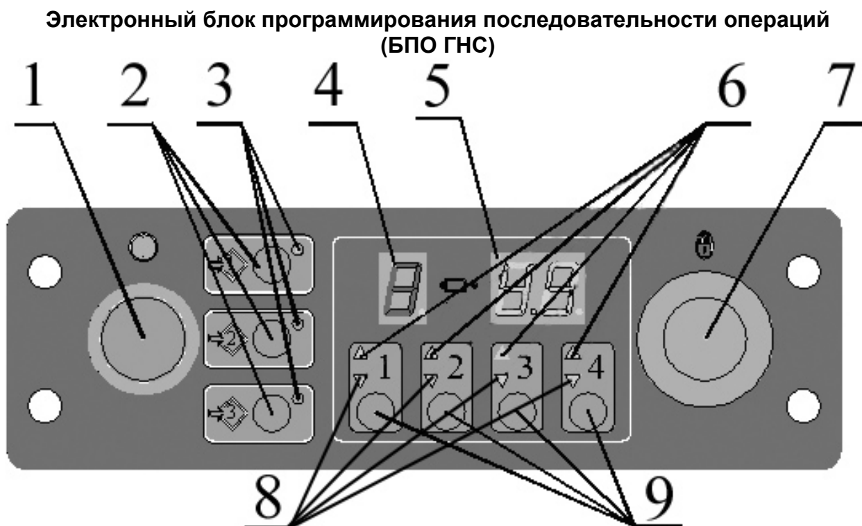
Рис.18 Панель блока программирования последовательности операций 1 — выключатель питания блока; 2 — кнопки отработки запрограммированных программ P1, P2, P3; 3 — сигнализаторы программ P1, P2, P3; 4 — сигнализатор номера работающей секции распределителя EHS; 5 — индикатор величины потока масла работающей секции; 6 — сигнализаторы подъема соответствующих секций распределителя EHS; 7 — выключатель «STOP» аварийного останова; 8 — сигнализаторы опускания соответствующих секций распределителя EHS; 9 — кнопки выбора секции распределителя EHS.
