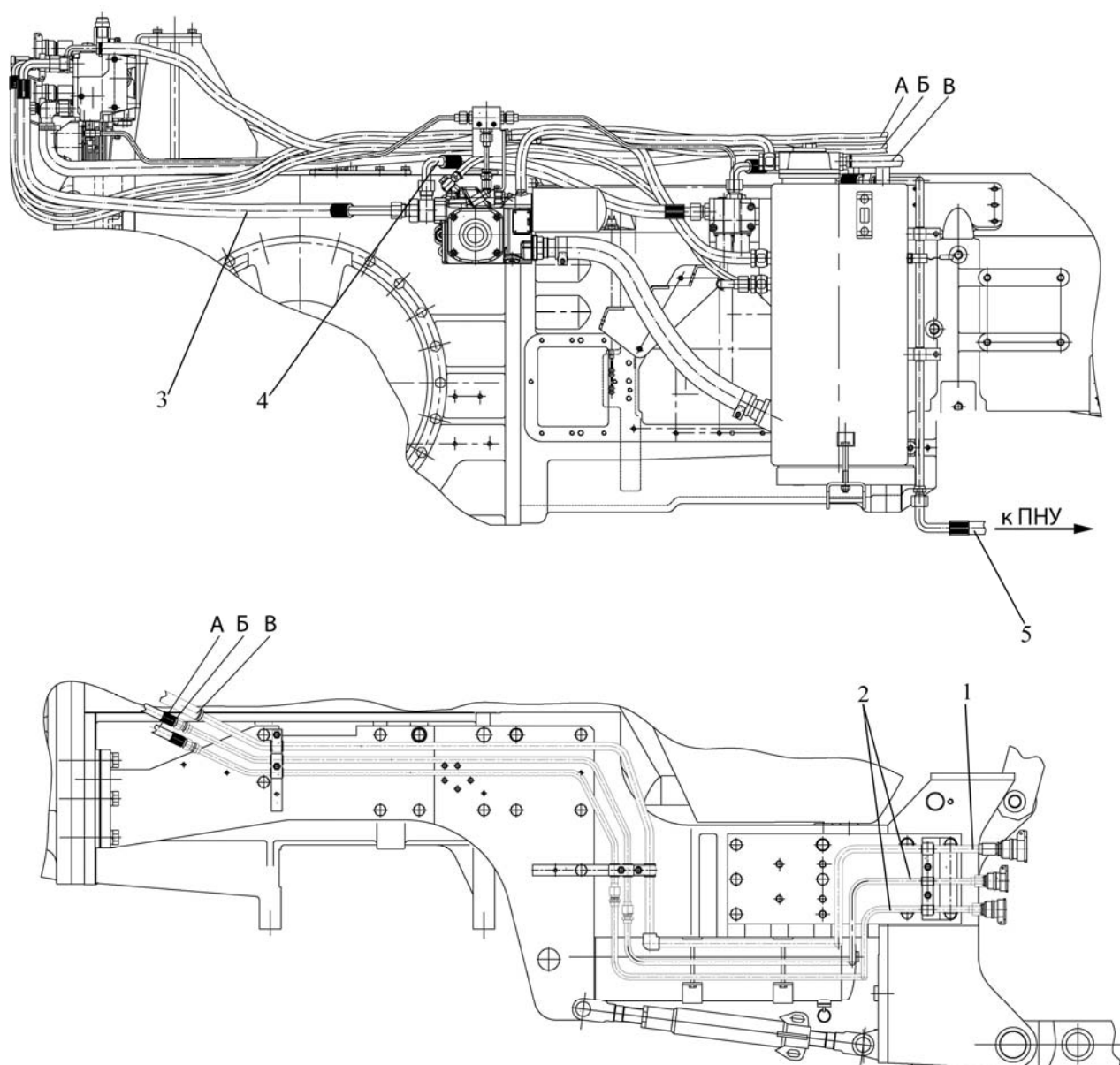
Рис.11 Компоновка узлов гидросистемы на тракторе (вид сбоку):
