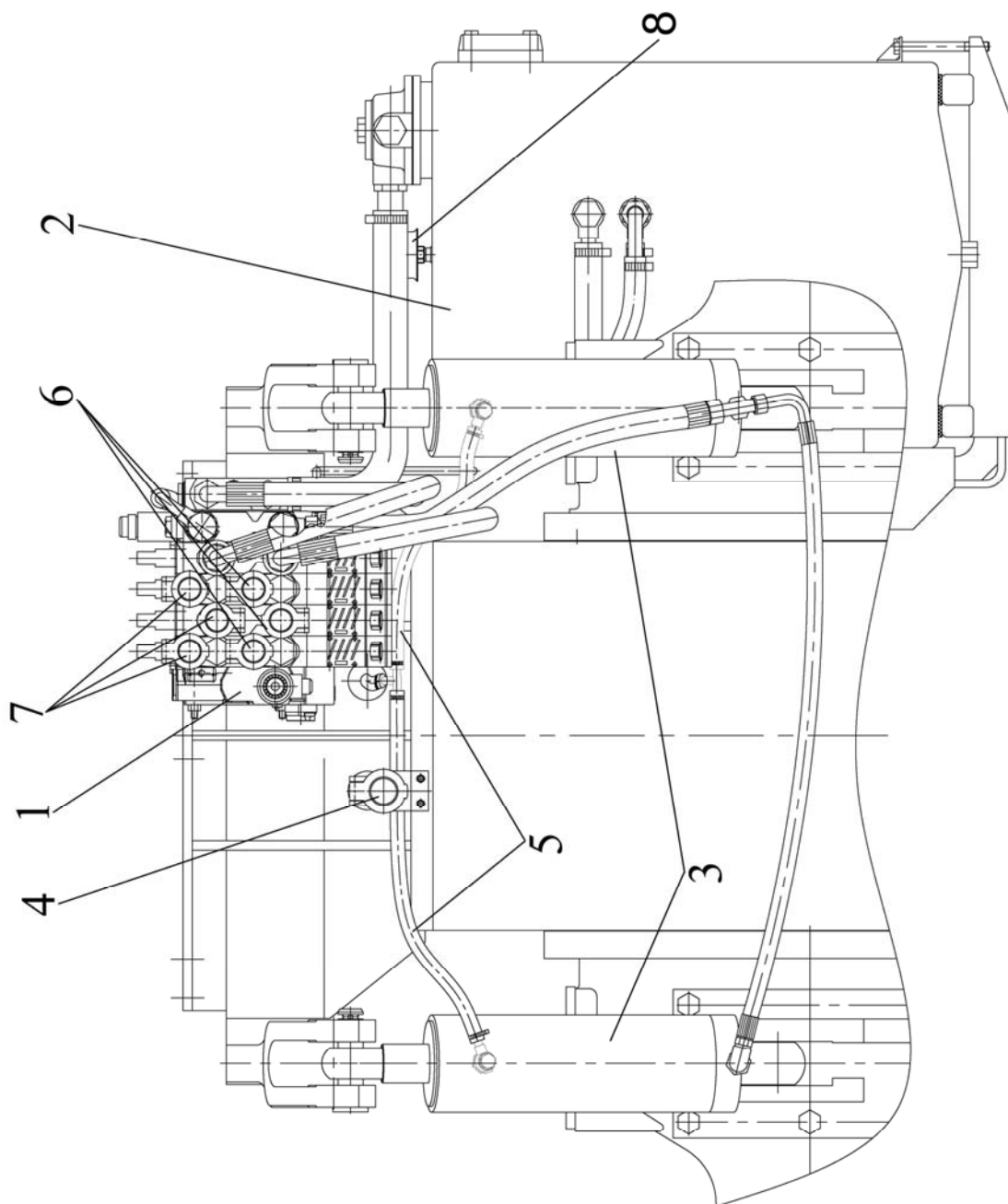
Рис.9 Компоновка узлов гидросистемы на тракторе (вид сзади):
