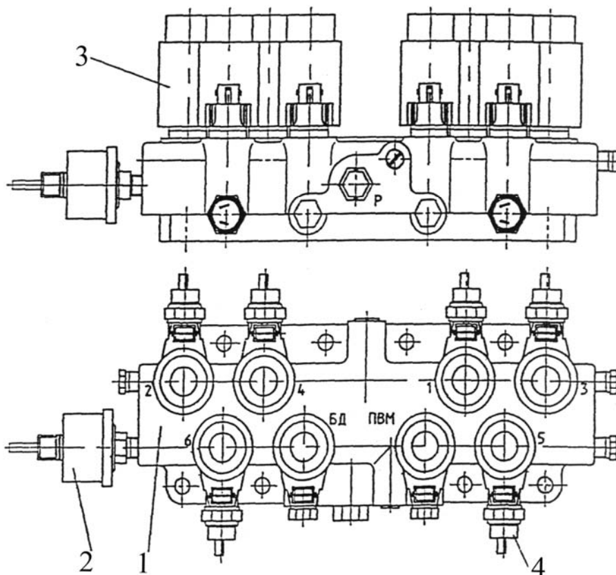
Рис. 27 Распределитель гидросистемы трансмиссии: 1 — корпус; 2 — датчик давления; 3 — электрогидрораспределитель; 4 — датчик давления.
