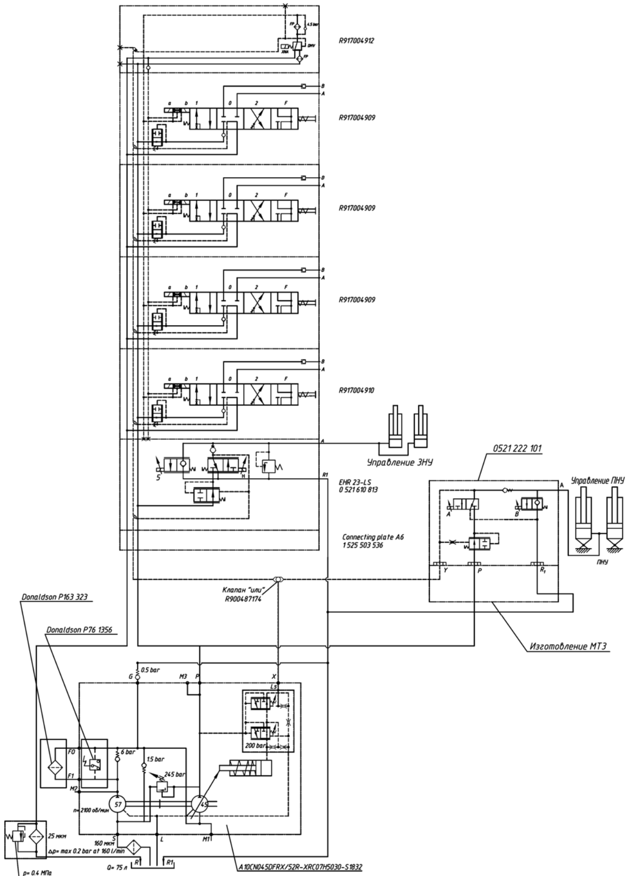
Рис.1а Схема принципиальная гидравлическая тракторов БЕЛАРУС-2522.1/2822.1/3022.1
