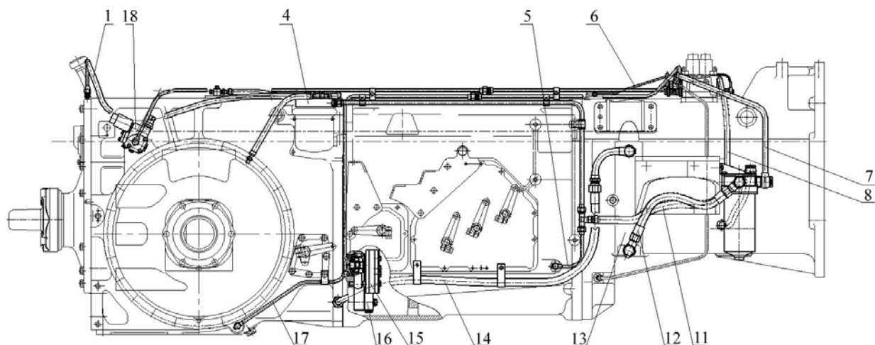
Рис. 24 Расположение элементов гидросистемы смазки трансмиссии (вид справа):
