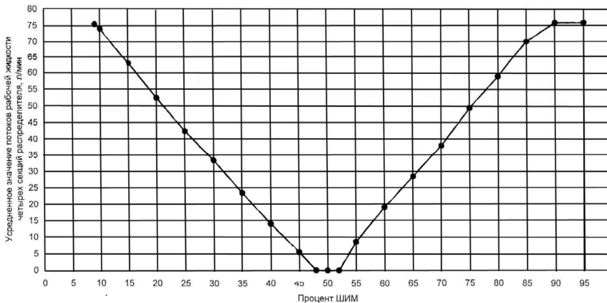
Рис.4. Зависимость потока рабочей жидкости на выходе из секций распределителя SB 23LS-EHS от величины управляющего сигнала при управлении электроджойстиком.
